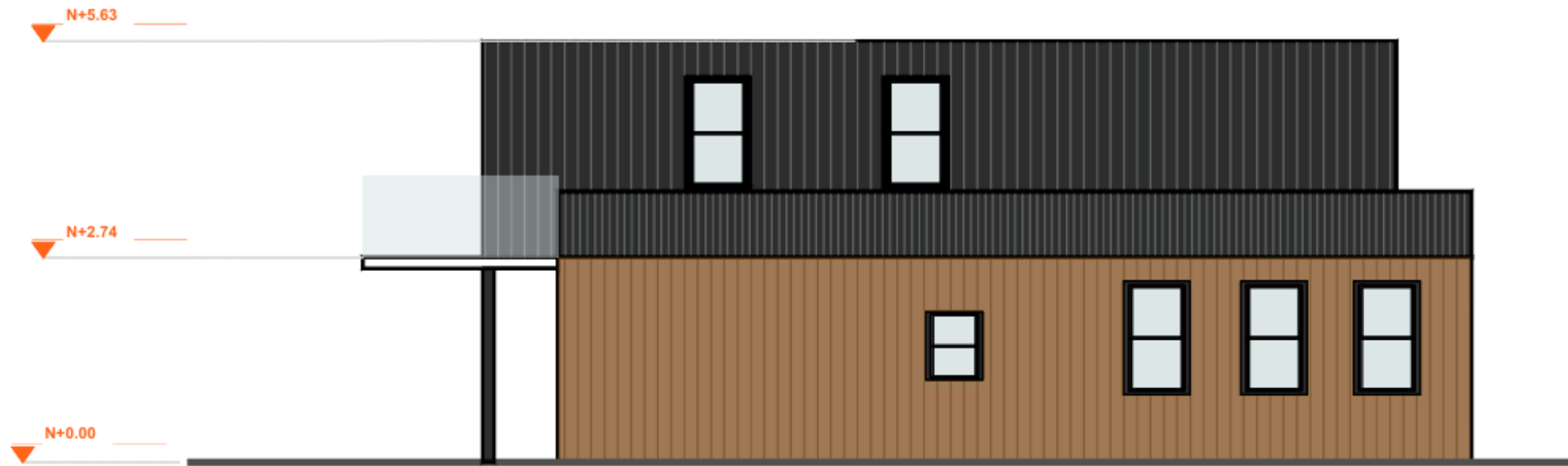
RIGTH ELEVATION
